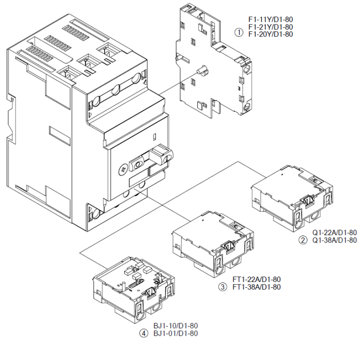
NDD1-80 配合附件
