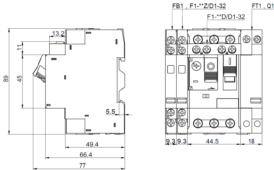
图 1 NDD1-32 断路器及配合侧挂附件的外形及安装尺寸
