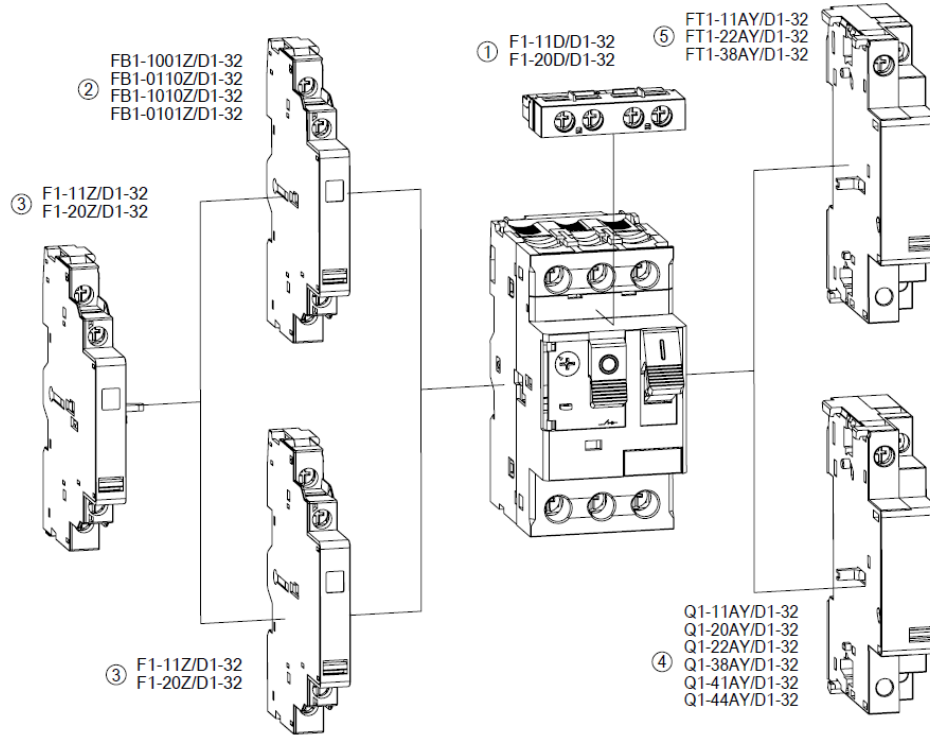
NDD1-32 配合附件
